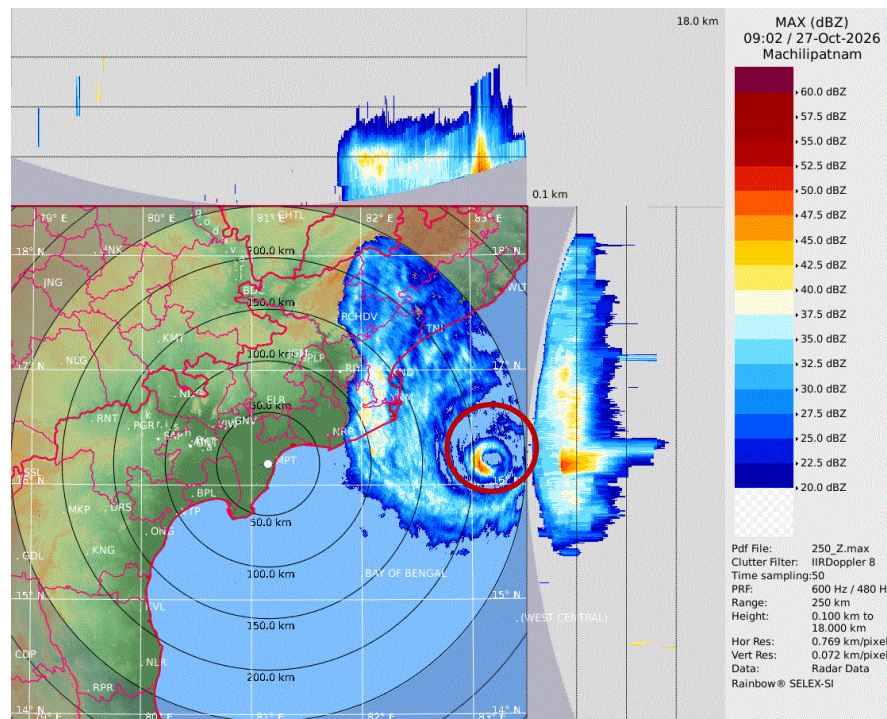
Radar Image of Machhliapatnam at 1430 hrs IST of 27 th Oct 2026
