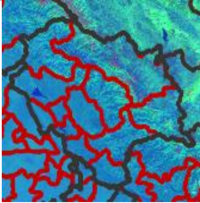
Satellite Image based on 11:15 IST
